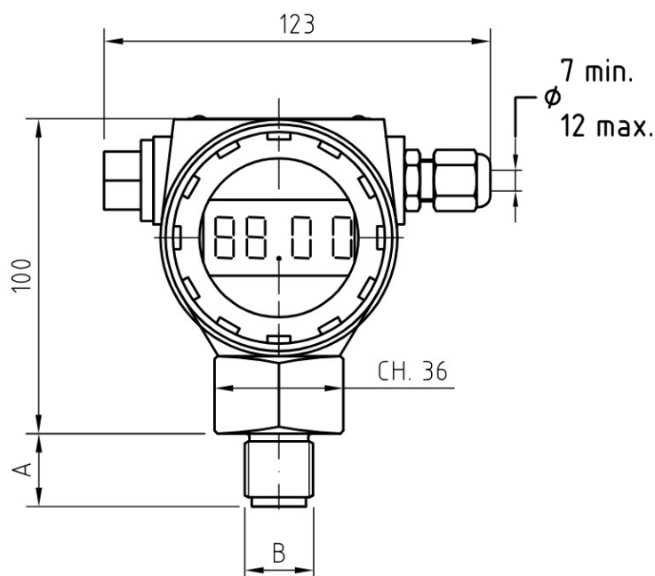
Figure 3 - Attacco filettato per Campo Nominale fino a 1000 bar Screwed connection for Nominal Range up to 1000 bar
