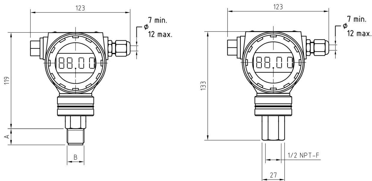
Figure 2 - Attacco filettato per Campo Nominale fino a 30 bar Screwed connection for Nominal Range up to 30 bar
